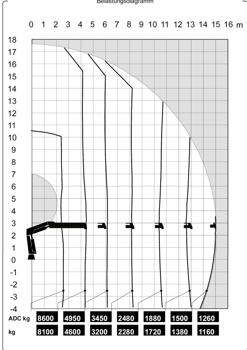
Belastungsdiagramm
