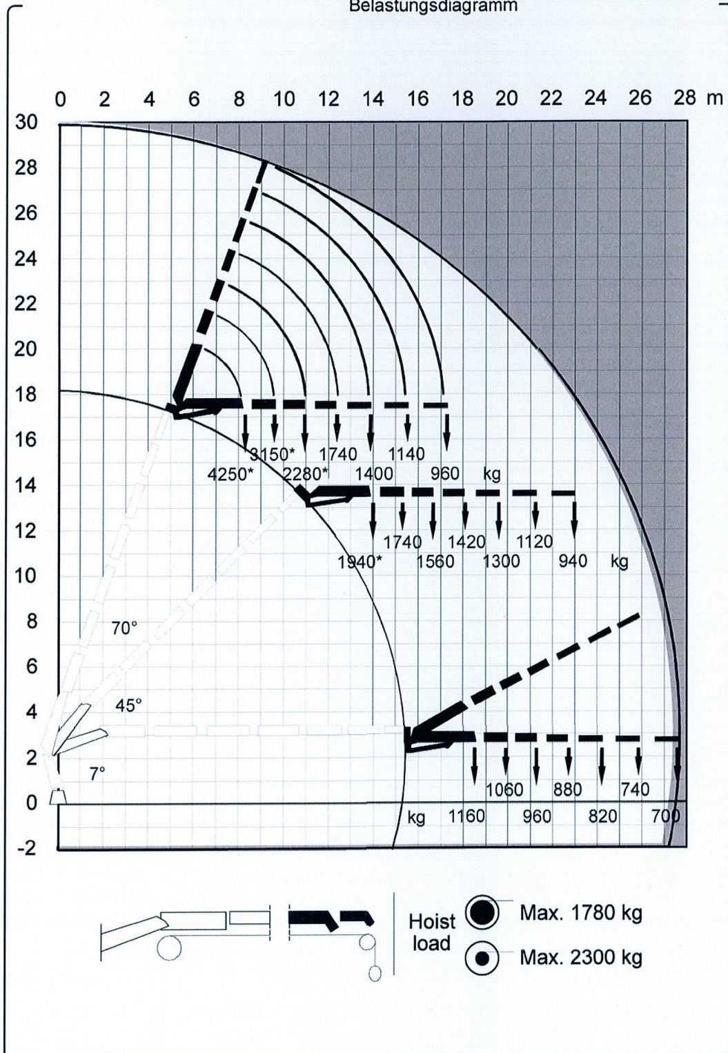
Belastungsdiagramm
